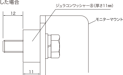
(図2) P3-M8×30アブセットボルトとジュラコンワッシャーを併用した場合
