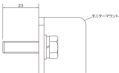
(図2) P3-M8×30アブセットボルトの場合
