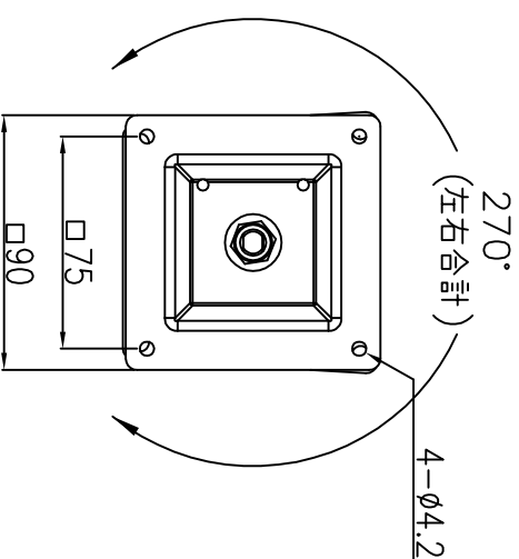
前図(正面)
