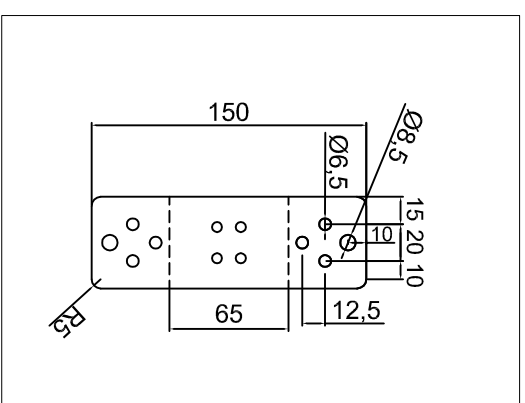
取付金具寸法
