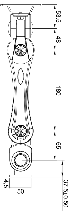
取付金具寸法
