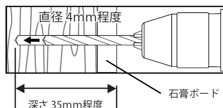
下穴は真っ直ぐに開けるよう注意を
