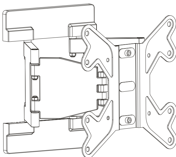
A テレビ金具本体
