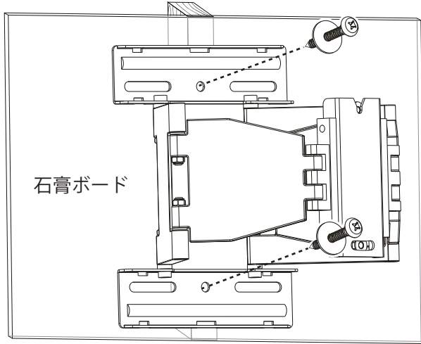
壁へのネジ打ち
