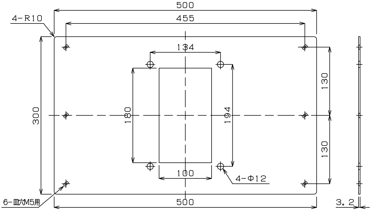
【HA-155補強金具A】 SPCC3.2t 2.5Y9/1半艶塗装
