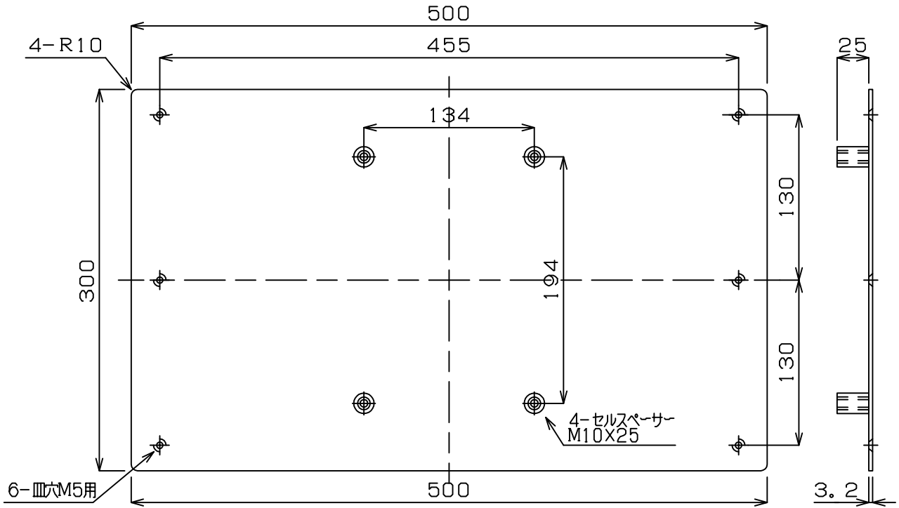
【HA-155補強金具B】 SPCC3.2t 2.5Y9/1半艶塗装
